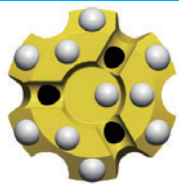
Type 53 (Ø70-Ø89)
